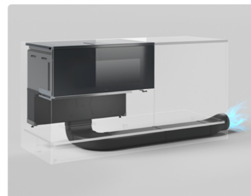
Odtah do boku Side outlet
