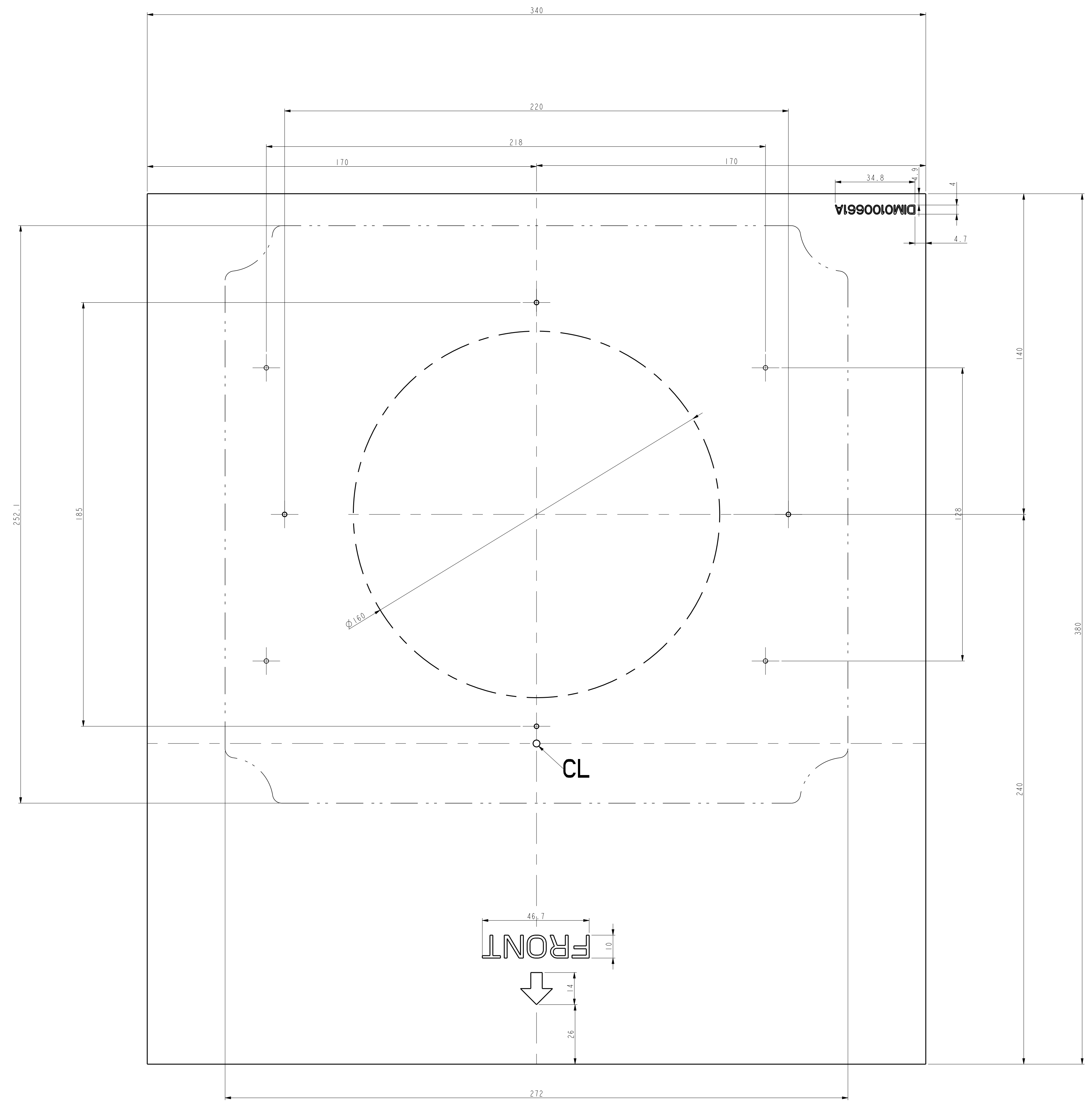
VISTA VALIDA PER LA VERIFICA DIMENSIONALE DELLA DIMA
